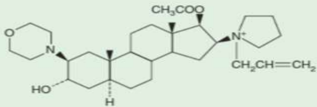
Rocuronium
